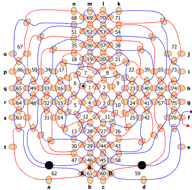
Skizze 1: Kopf Teil 1
