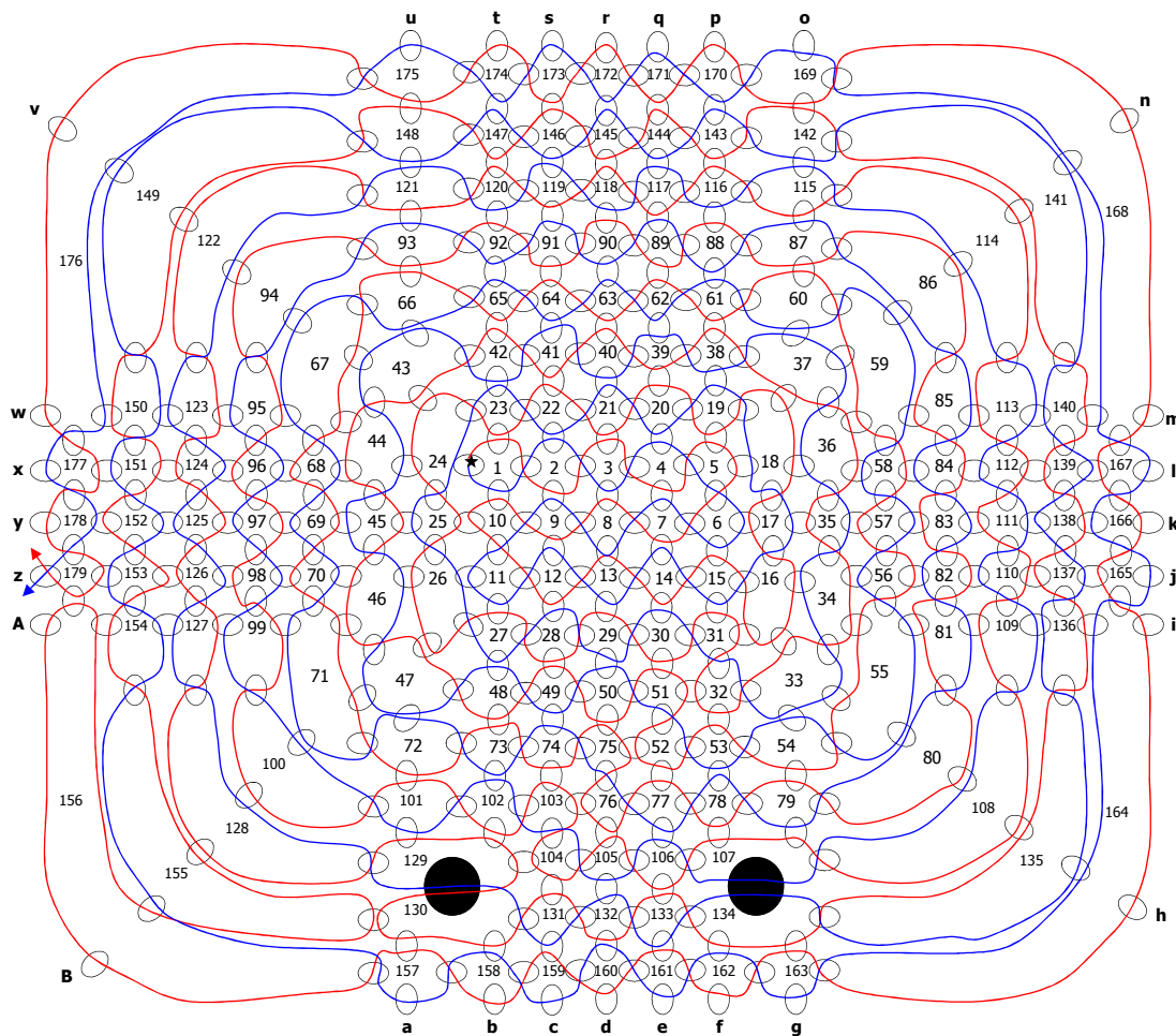
Skizze 1: Kopf Teil 1
