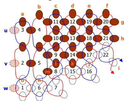
Skizze 5: Flügel Vorderseite
