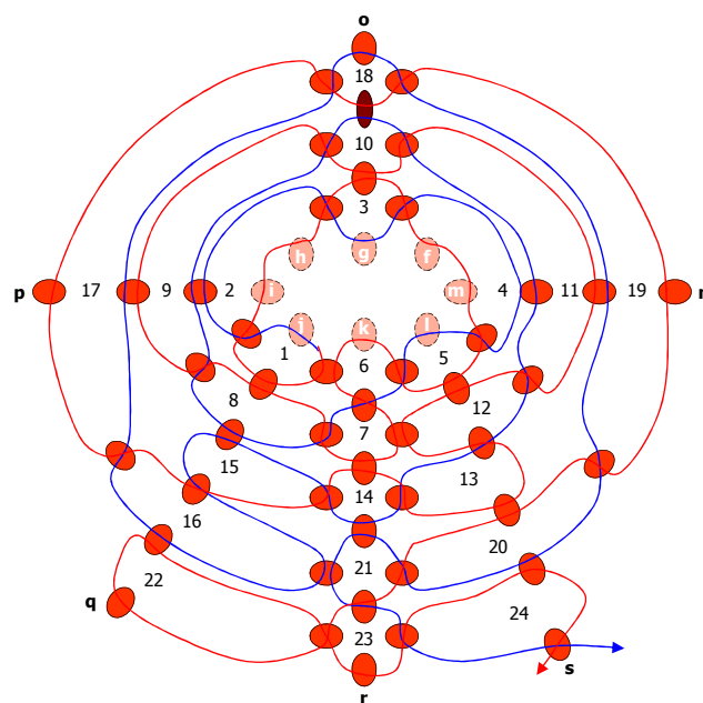
Skizze 13: Schwanz Teil 1
